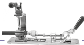
Montagegerät 611050G
