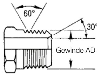
ØA Abmessungen werden an der 4. Gewindespitze gemessen
